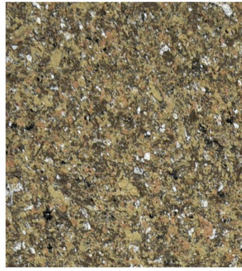
332 Landslide
